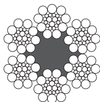
6x22 (9/12-Δ)FS+Органический сердечник
